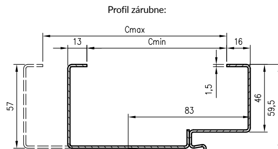
Profil zárubne:
