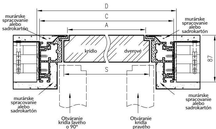
Priečný prierez dverí 50 mm s obráteným falcom – otváranie smerom dovnútra
