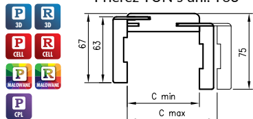
Prierez TUN s uhl. T63
