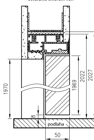
Zvislý prierez dverí 50 mm bezfalcové – otváranie smerom von
