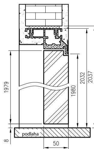
Zvislý profil dverí 50 mm s obráteným falcom – otváranie smerom dovnútra
